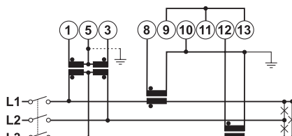
Fig. 12 AV6
