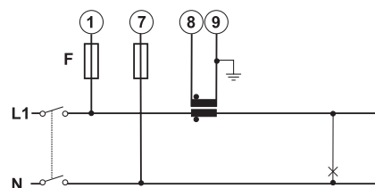
Fig. 20 AV5, AV6
