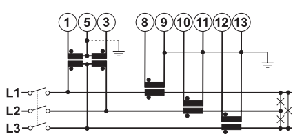
Fig. 11 AV6
